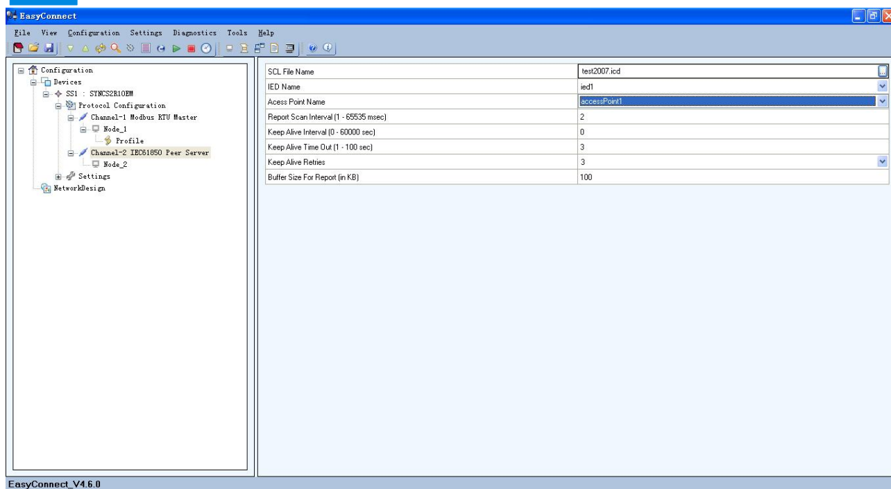
图 36 IEC61850 通道属性配置举例
