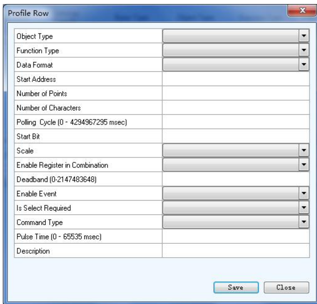
图 31 属性编辑
