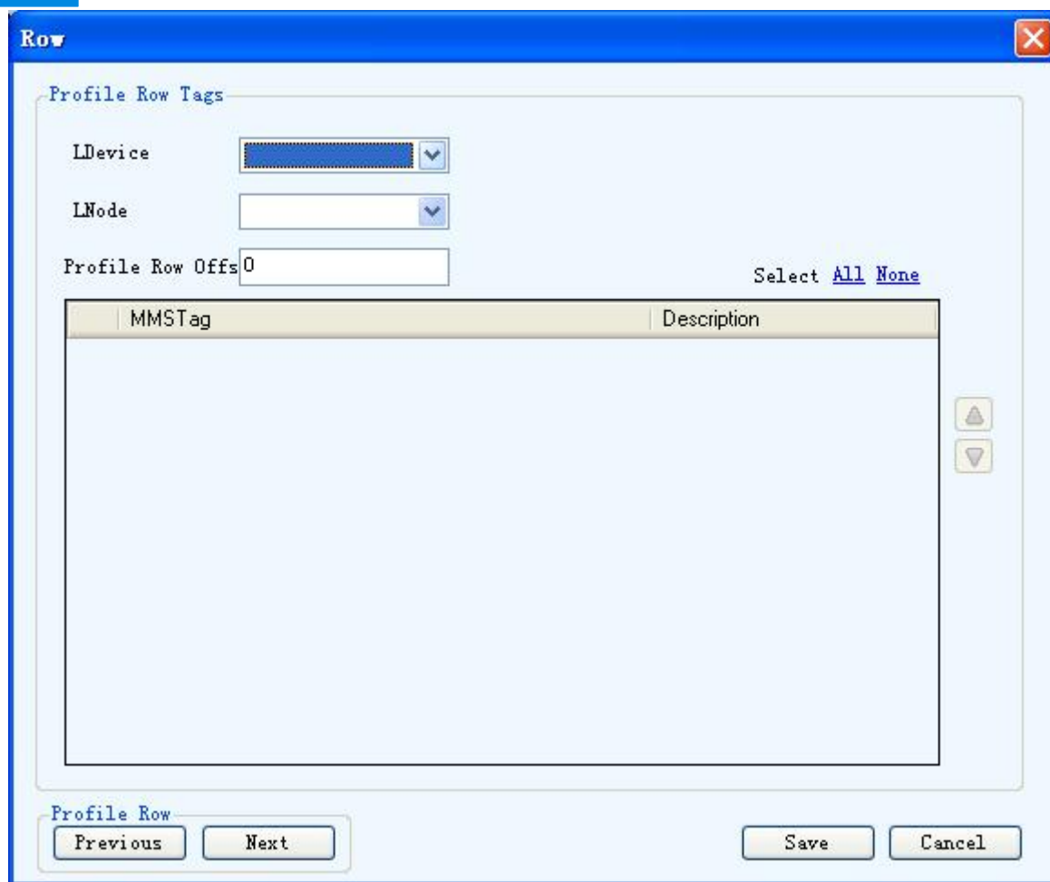
图 39 映射参数
