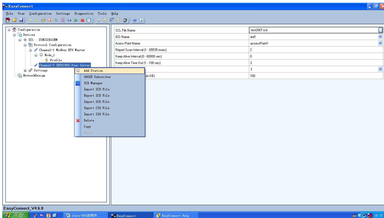
图 37 IEC61850 通道添加节点
